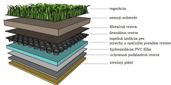
Schéma vegetačnej strechy
