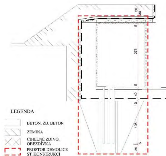
Obr. 3 Schematický řez objektem
