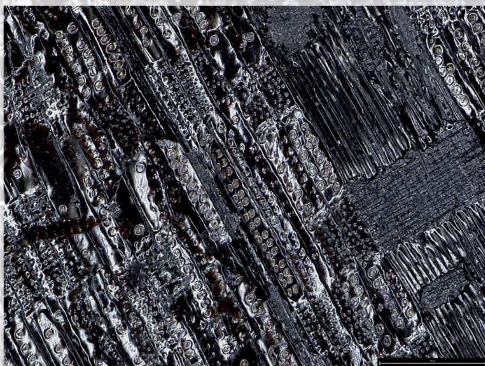
Biochar – drevené uhlie si stále zachováva štruktúru pôvodnej dreviny, na obrázku smrekovec opadavý ( Larix decidua ) v radiálnom reze, 1000x zväčšenie, Leica DVM6 M, (foto: Š. Heřmánková)
