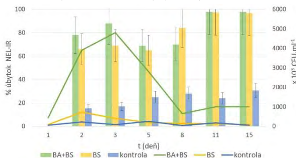
Obr. 1 Degradácia RL (NEL-IR) kombinovaným prístupom BA+BS a samotnou BS; vývoj koncentrácie baktérií – CFU.ml -1 počas biodegradácie.
