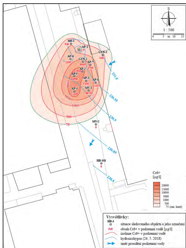
Obr. 1 Stav kontaminace saturované zóny Cr^{6+} v dané oblasti před zahájením plnoprovozní sanace
