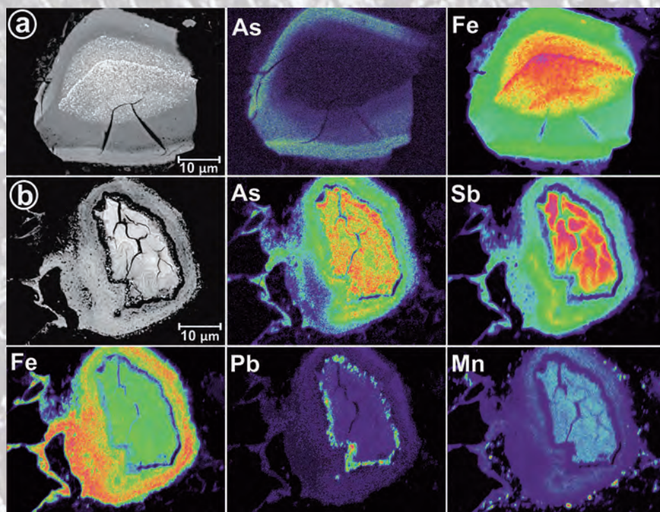
BSE snímky sekundárných oxidov Fe s komplikovanou zonálnou stavbou v: a) zmesi pôda-elektársky popol bohatej na As (Zemianske Kostoľany) a b) iniciálnej pôde s vysokým obsahom Sb a As z banskej oblasti (Poproč) s príslušnými distribučnými mapami vybraných chemických prvkov (Hiller et al. 2021, DOI: 10.1016/j.envpol.2021.117268)
