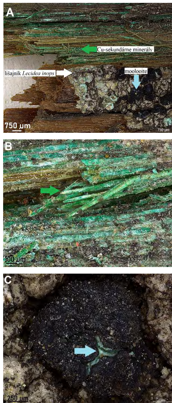
Obr. 2 Mikrofotografie A – lišajníka Lecidea inops na suchom dreve prerastenom zelenými sekundárnymi minerálmi medi. B – detail zelených sekundárnych minerálov medi. C – detail na tyrkysovomodrú depozíciu minerálu moolooit v plodničke lišajníka L. inops
