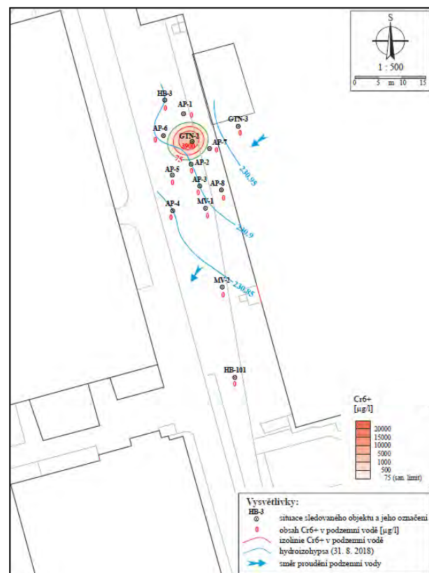
Obr. 2 Stav kontaminace saturované zóny Cr^{6+} 3 měsíce po aplikaci
