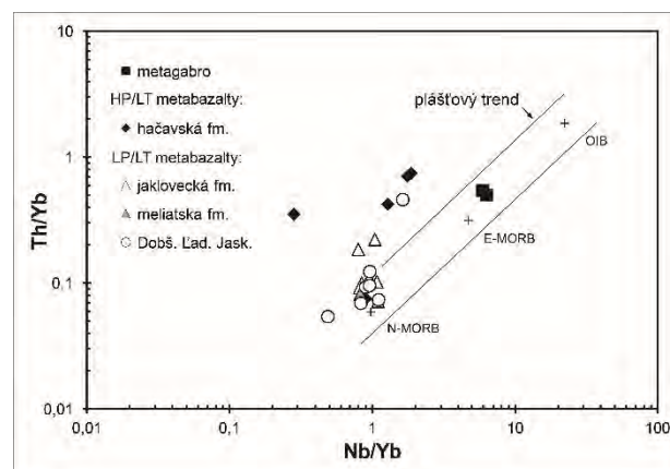
Obr. 3 Metagabrá z hačavskej formácie v diagrame Nb/Yb vs. Th/Yb v porovnaní s metabazaltami rôznych meliatikových formácií. Ich geochemická blízkosť typu E-MORB ich odlišuje od ostatných metabazitov meliatika, ktoré sú blízke oceánskeho typu N-MORB alebo horninám ostrovných oblúkov
