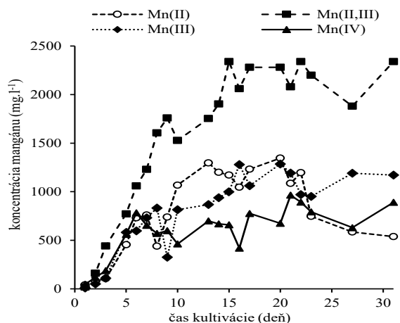
Obr. 1 Zmeny koncentrácie celkového rozpusteného mangánu v živnom médiu počas statickej kultivácie mikroskopickej vláknitej huby A. niger v prítomnosti rôznych oxidov mangánu
